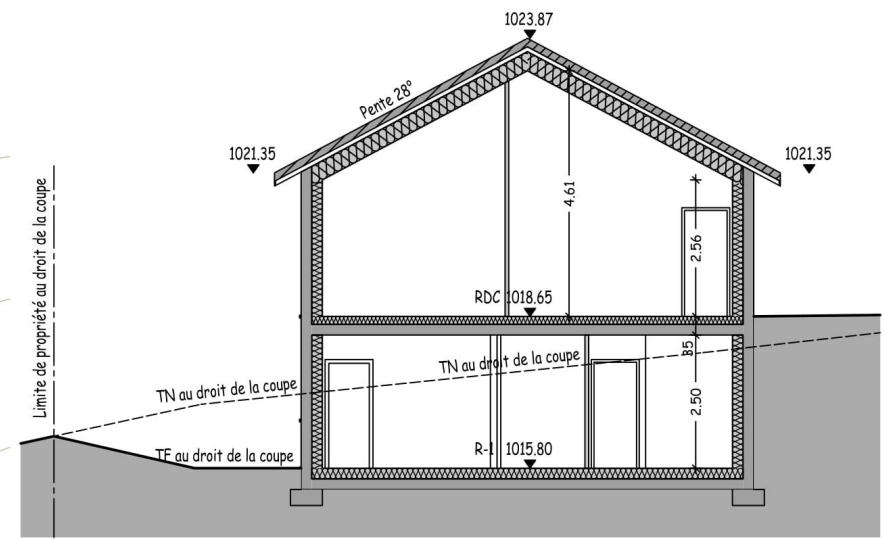
COUPE DE PRINCIPLE C - 1/100e
