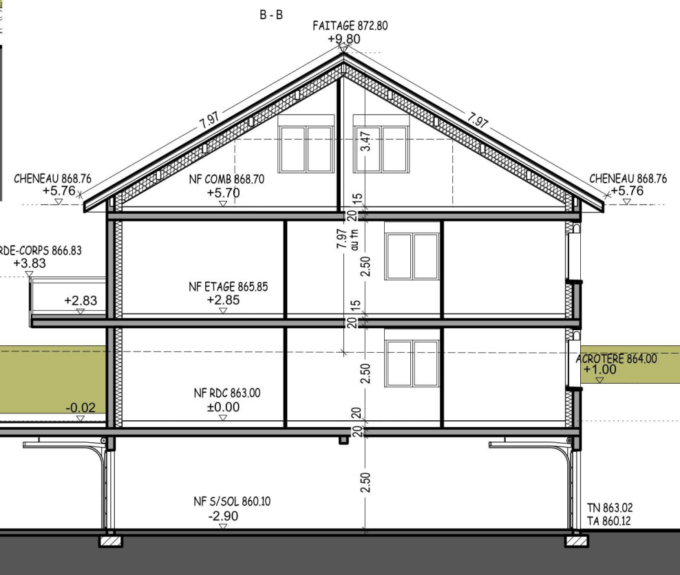
COUPE B 1/100°
