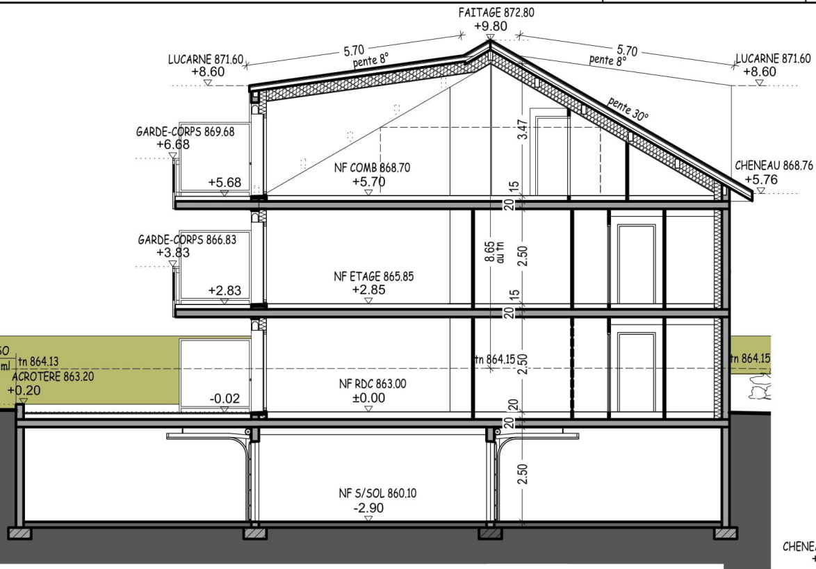
COUPE A 1/100°
