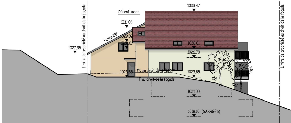
FACADE NORD-OUEST - 17 logements
