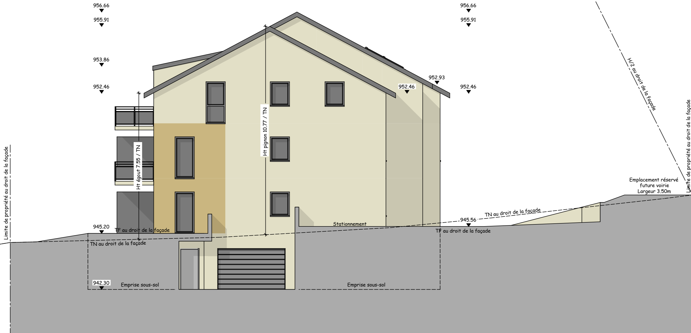
PC05 - FACADE NORD EST - 1/100e
